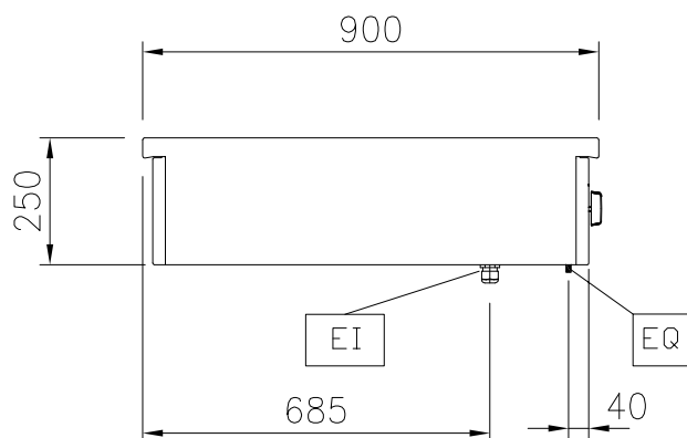
Zij aanzicht
